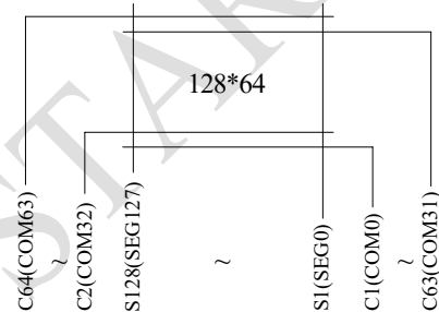
SEG & COM Layout
